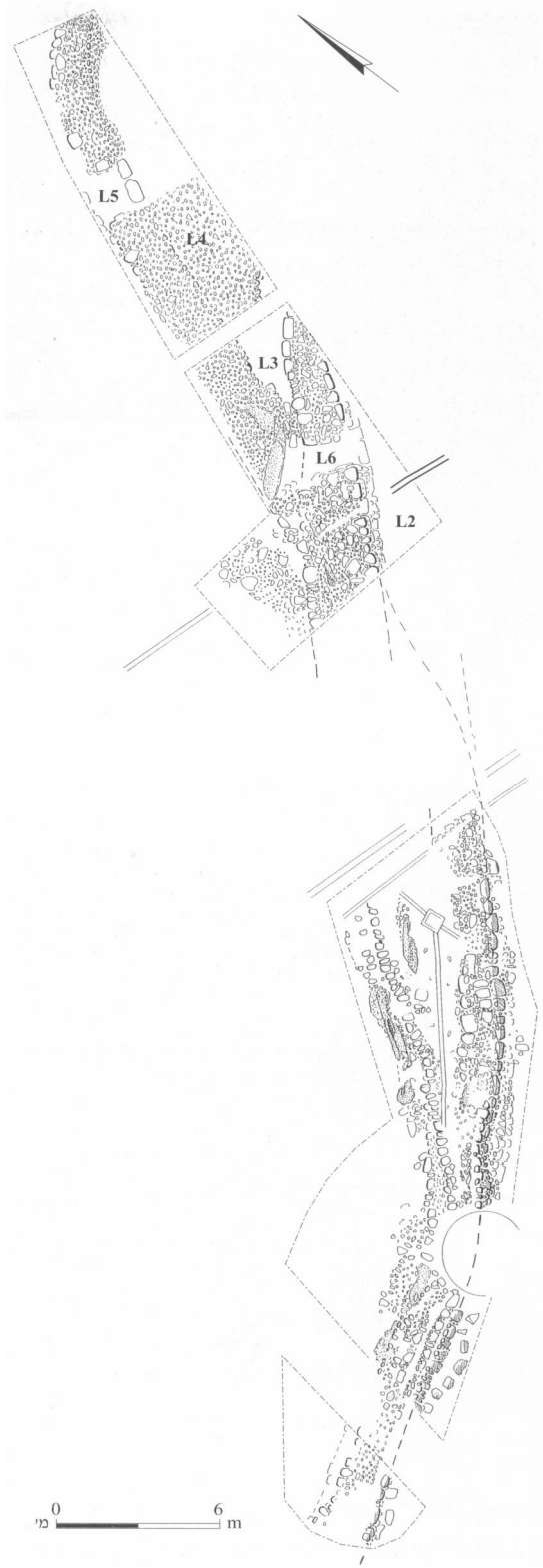
תכנית 2. אמת המים בשטח A2: קטע 6.
